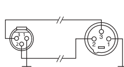
Schéma électrique Schema elettrico
